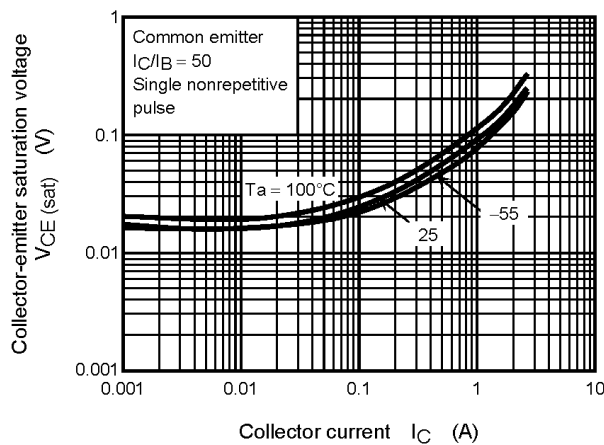
Fig. 7.3 V_{CE(sat)} - I_C
