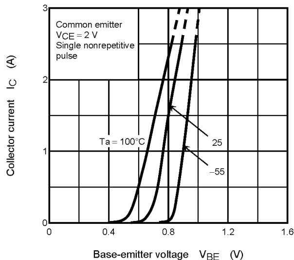
Fig. 7.5 I_C - V_{BE}
