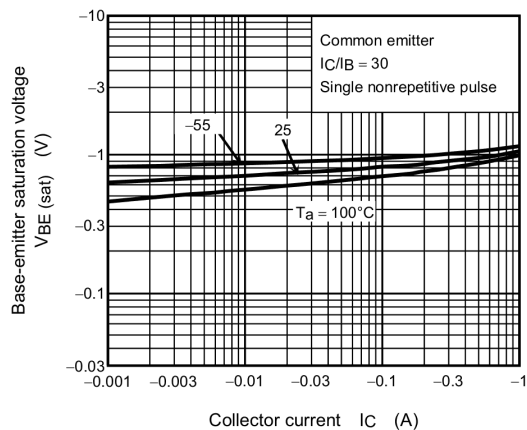
Fig. 7.4 V_{BE(sat)} - I_C
