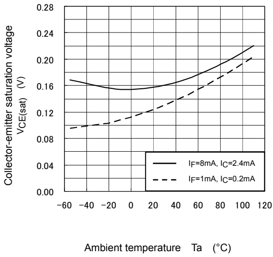
V_{CE(sat)} - T_a
