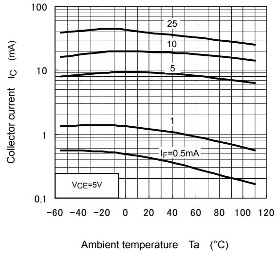
I_C - T_a
