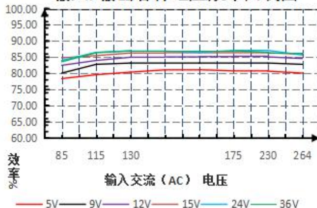
输入/输出各种电压效率曲线图
