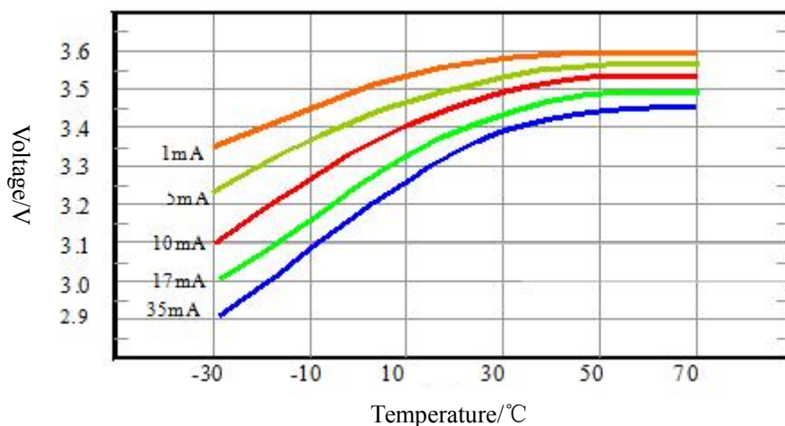
不同温度下电压平台特性图
