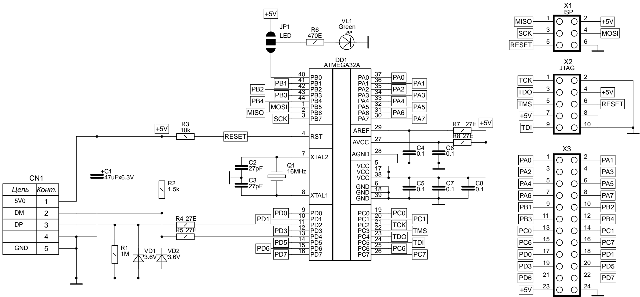
USB-ATMEGA
