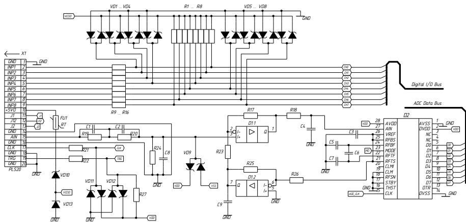
Электрическая принципиальная схема входных цепей прибора "LOGIC-U PRO"
